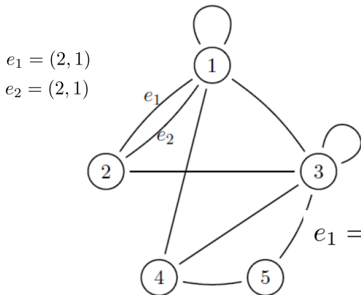
Grafo não orientado
